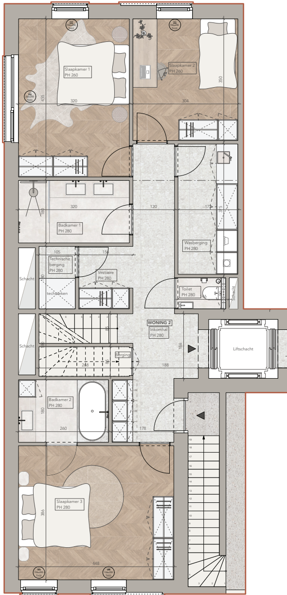
Grondplan LOFTWONING 2
